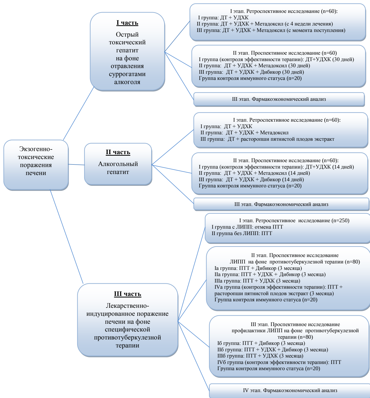
Рис. 1. Дизайн исследования
